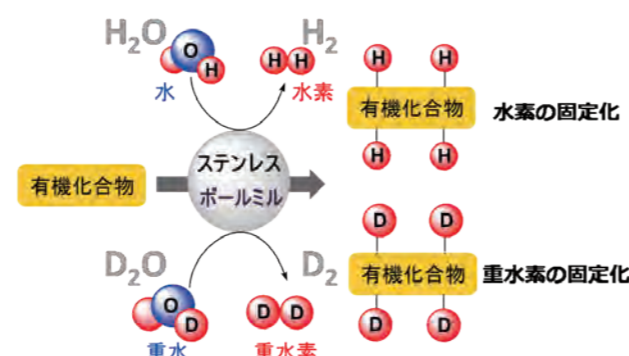
水から水素を取り出す・水を還元剤とした接触還元
