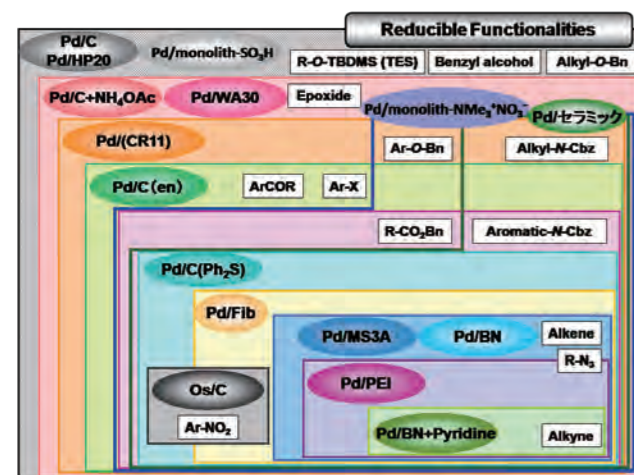
当研究室で開発・実用化された官能基選択的触媒
